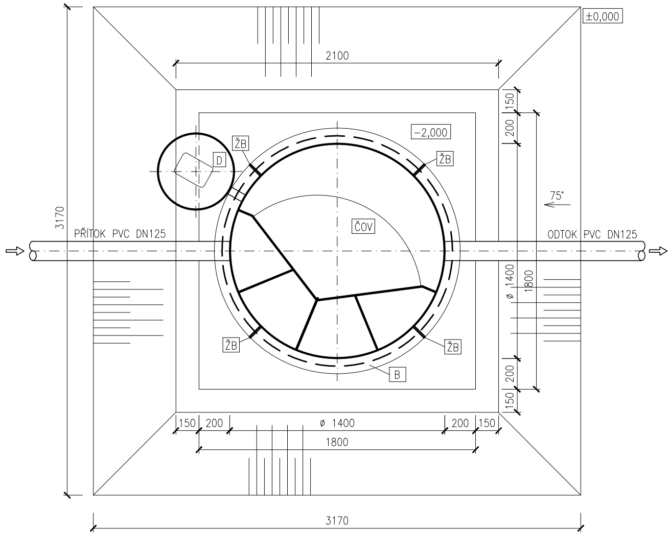
Půdorys
